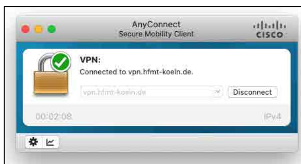
Abbildung 24: Disconnect
